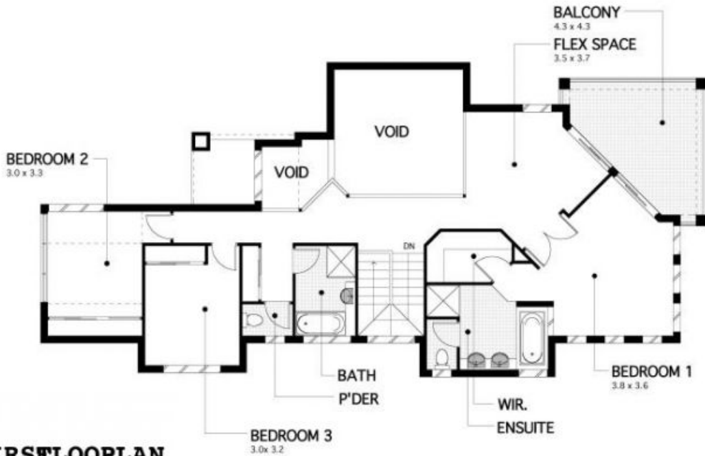
FIRSELOORLAN
